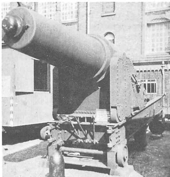
29 cm (11 tommers) riflet forladekanon. Støbt 1868. Stod på Trekroner fra 1869 til 1898. Samlet vægt 37 tons. Største skudvidde 7000 m
