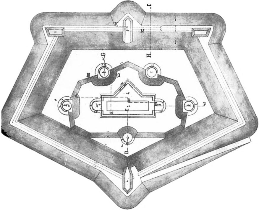
HORIZONTALT SNIT.
